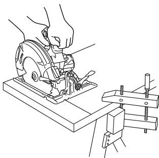
EXEMPLE TYPE DE SOUTIEN MANUEL DE LA SCIE ET, SOUTIEN LA PIÈCE ET D'ACHEMINEMENT DU CORDON.
